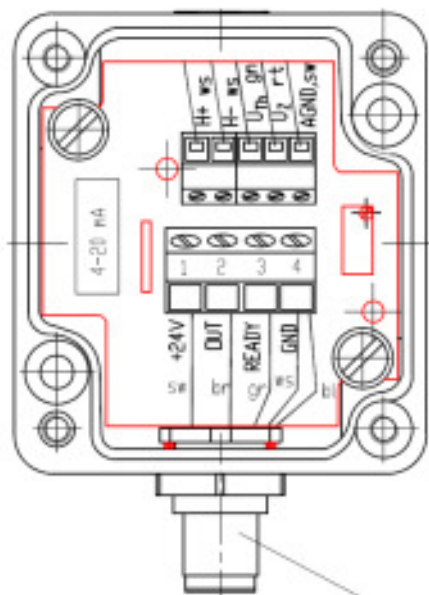
Einbaustecker 5-polig
